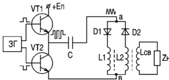
Рис. 2. Структурна схема діодного контуру
