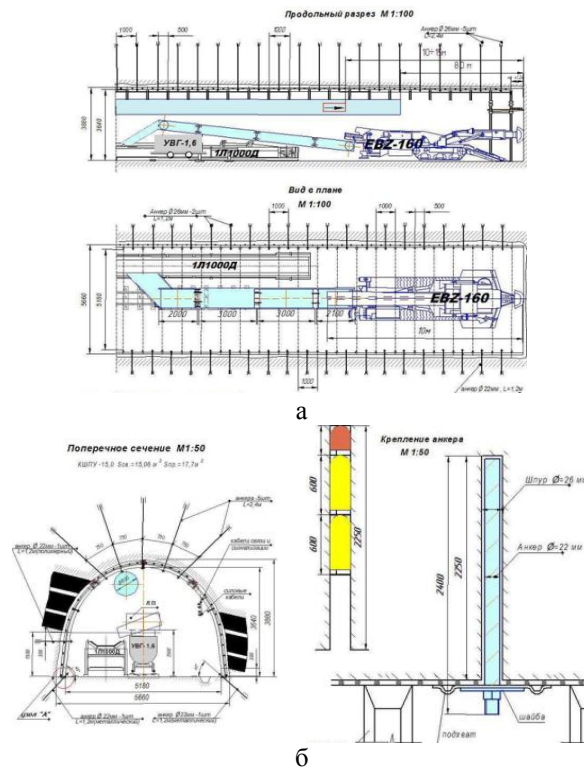
Рис. 2. Технологічна схема проведення (а), перетин та параметри кріплення (б) штреку з комбайном EBZ-160
