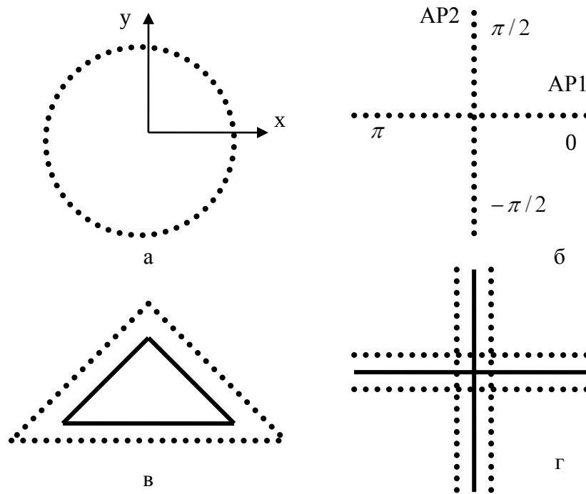
Рис. 1. Основні варіанти конфігурації АР кореляційно-інтерферометричних радіопеленгаторів: а – кільцева; б – система з двох ортогональних лінійних АР; в – трикутна з екрануванням; г – система з двох ортогональних лінійних АР з повним екрануванням
