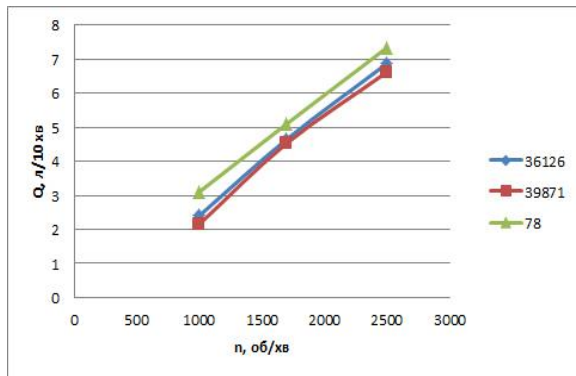
Рис. 1. Залежність витрати палива від частоти обертання колінчастого валу двигуна
