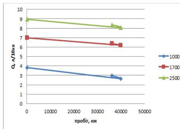
Рис. 4. Залежність витрати біодизеля від пробігу двигуна від початку експлуатації (або після капітального ремонту)
