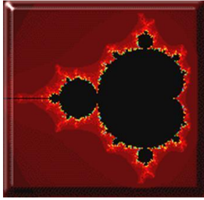
Рис. 4. Множина Мандельброта
