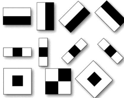
Рис. 1. Ознаки Хаара
