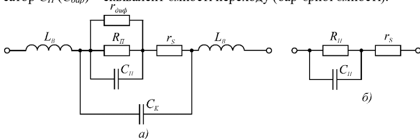
Рис. 1. Еквівалентні схеми варикапу [1, 2]:
