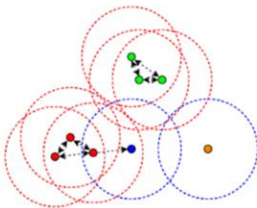
Рис. 1. Ілюстрація алгоритму DBSCAN
