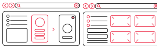
Рис. 1. Вигляд UX-дизайну
