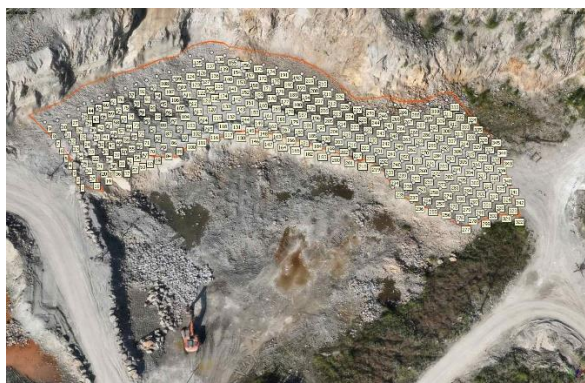
Рис. 2. Розташування свердловин в паспорті буровибухових робіт на Березівському-1 родовищі граніту
