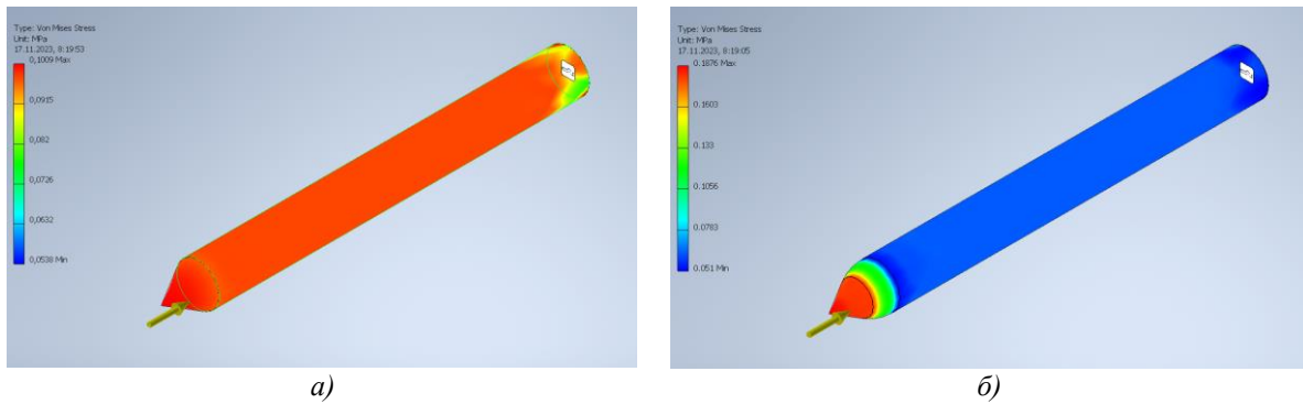
Рис.2. Результат моделювання напружень, що виникають при роботі конічної піки у звичайному виконанні (а) та при роботі піки зі значенням заокруглення основи у 111 мм (б)
